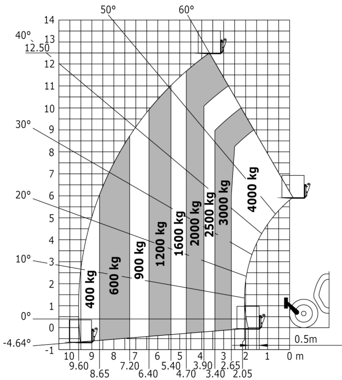
Makina lastik üzerinde çatal ile
